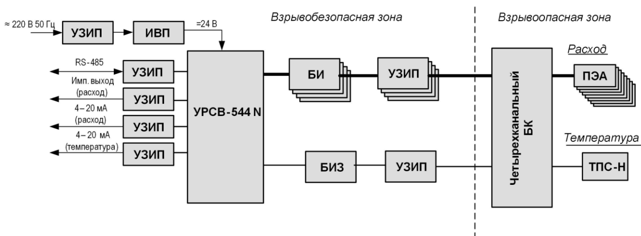
б) четырехлучевое исполнение расходомера
