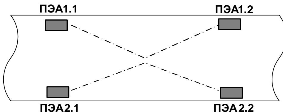
Рис.5. Положение пар ПЭА для V-схемы при размещении их в одной продольной плоскости (двухлучевое зондирование). Вид сверху.
