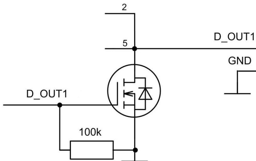
Рис.А.4. Схема оконечного каскада импульсного выхода.
