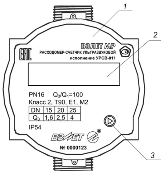
Вид сверху
