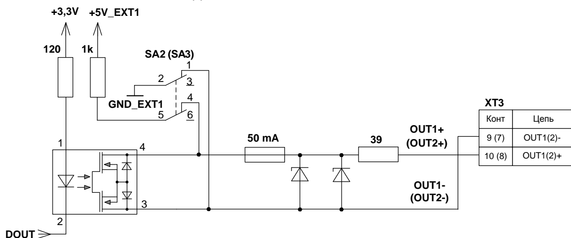
Рис.Б.1. Схема оконечного каскада универсальных выходов.
