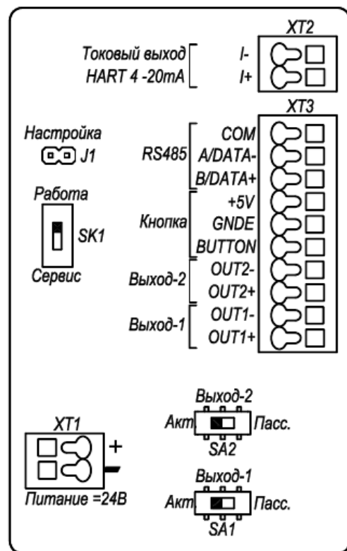
б) вид наклейки на задней крышке
