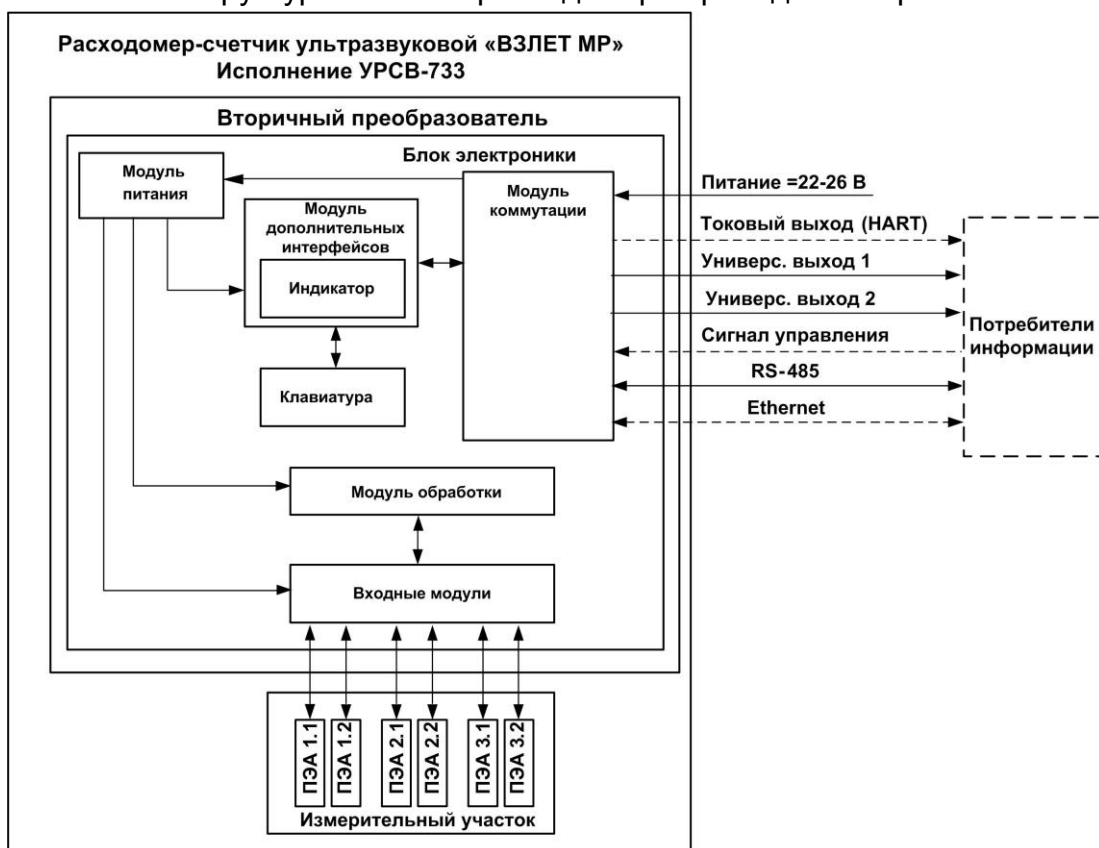
Рис.2. Структурная схема расходомера 3-х лучевого исполнения.
