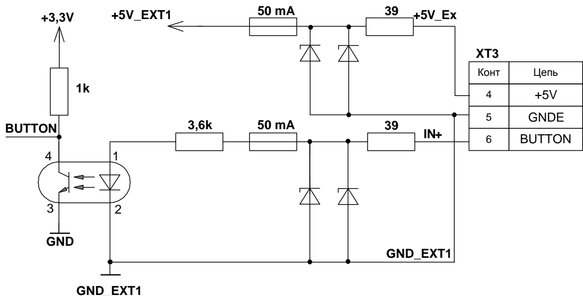
Рис.Б.3. Схема входного каскада расходомера.
