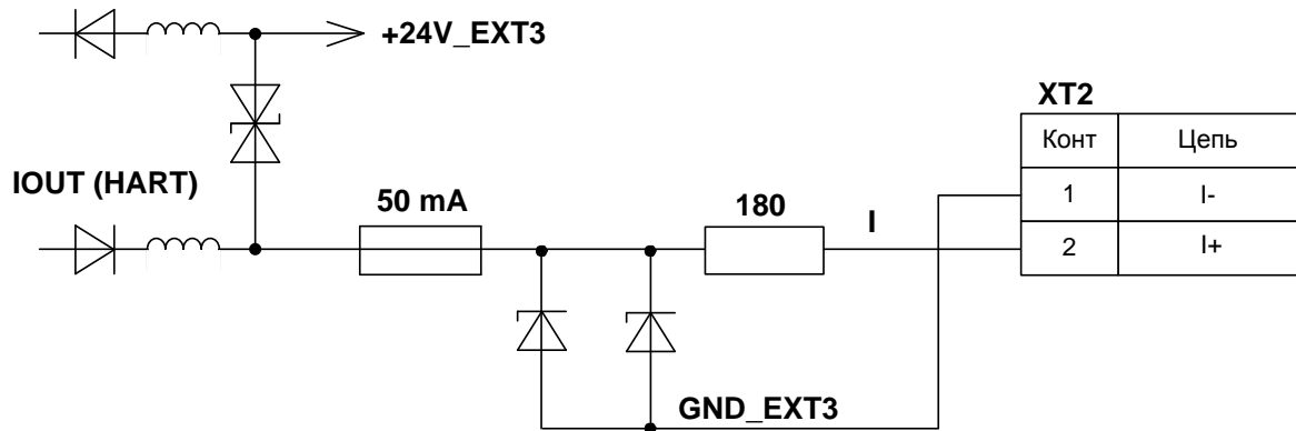
Рис.Б.2. Разъем токового выхода расходомера с HART-интерфейсом.
