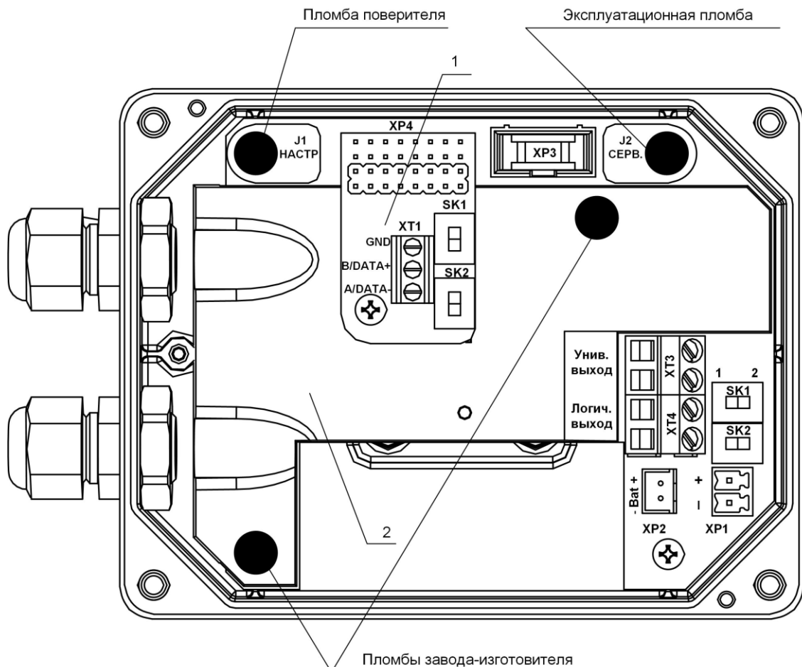
Рис.4. Вид вторичного преобразователя с модулем RS-485 (крышка снята).
