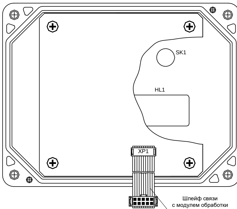
Рис.А.5. Вид модуля индикации с индикатором в прозрачной крышке вторичного преобразователя.
