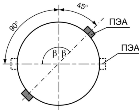
Рис.4. Рекомендуемые положения ПЭА при установке расходомера.
