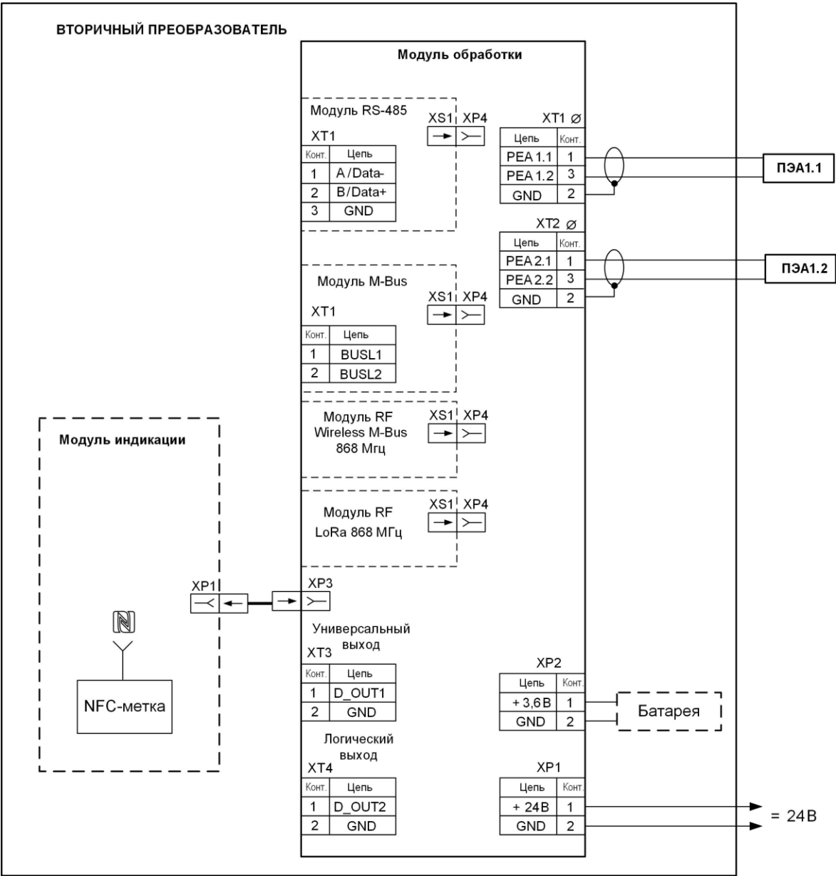
Рис.Б.1. Схема соединений расходомера УРСВ-311.
