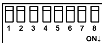
Рис.1. Блок микропереключателей адаптера.
