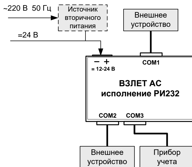
Рис.2. Общая схема подключения к адаптеру.
