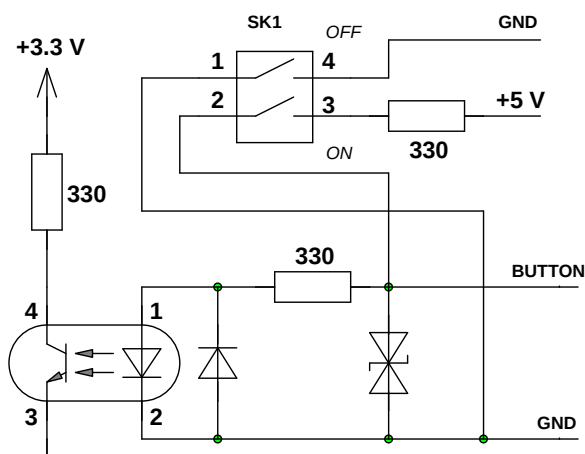
Рис.Б.3. Схема входного каскада расходомера.
