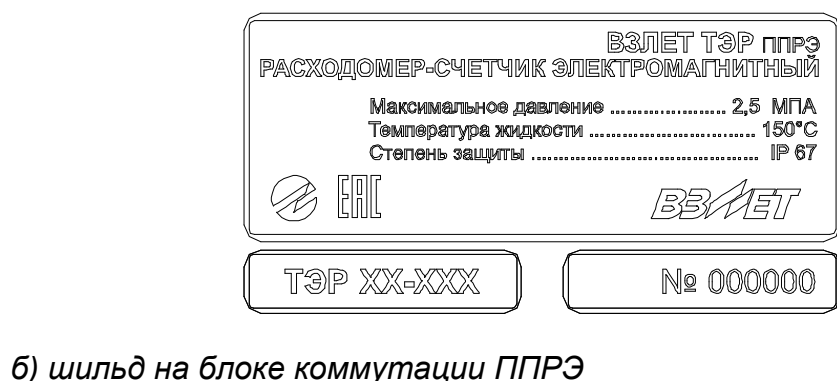
Рис.4. Вид шильдов расходомера в разнесенном конструктиве.
