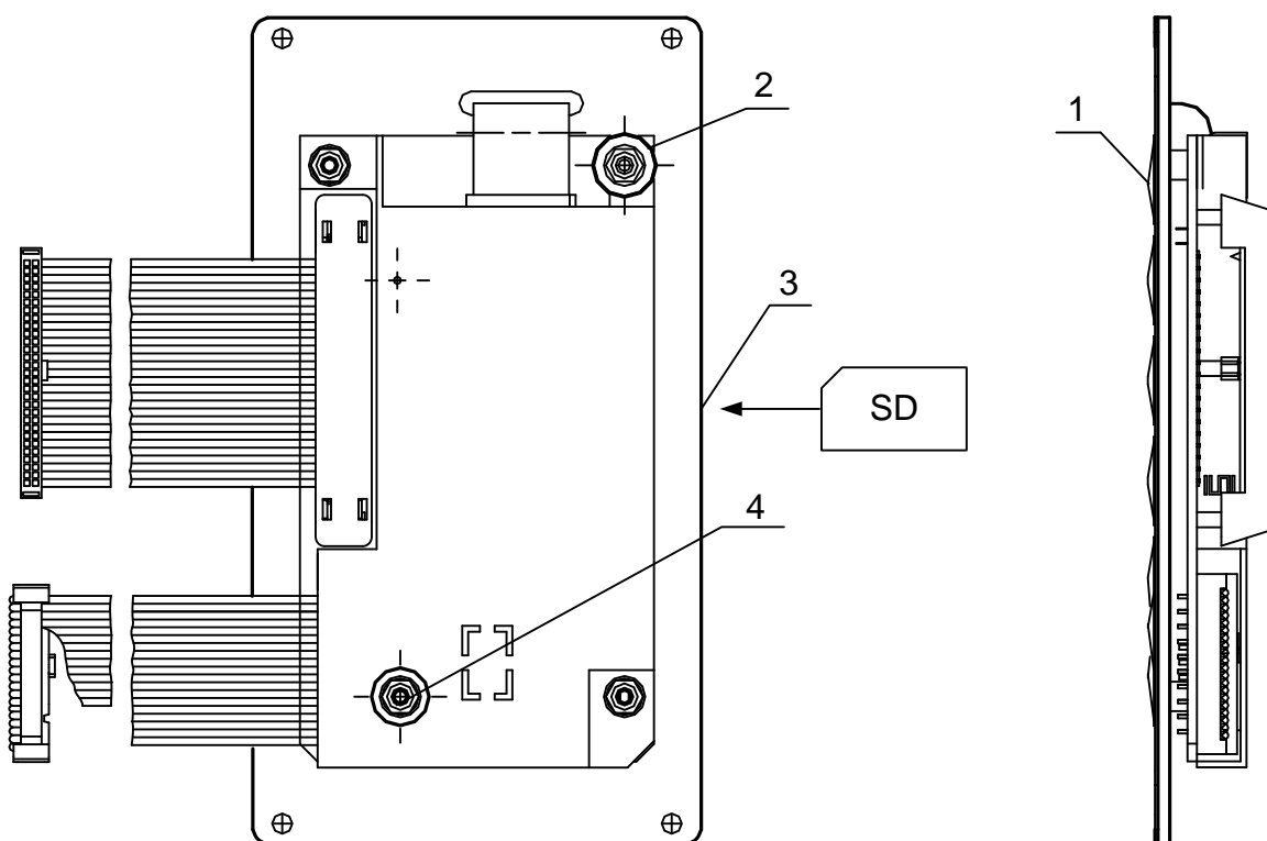
Рис.А.5. Преобразователь электроакустический ПЭА Н-222.
