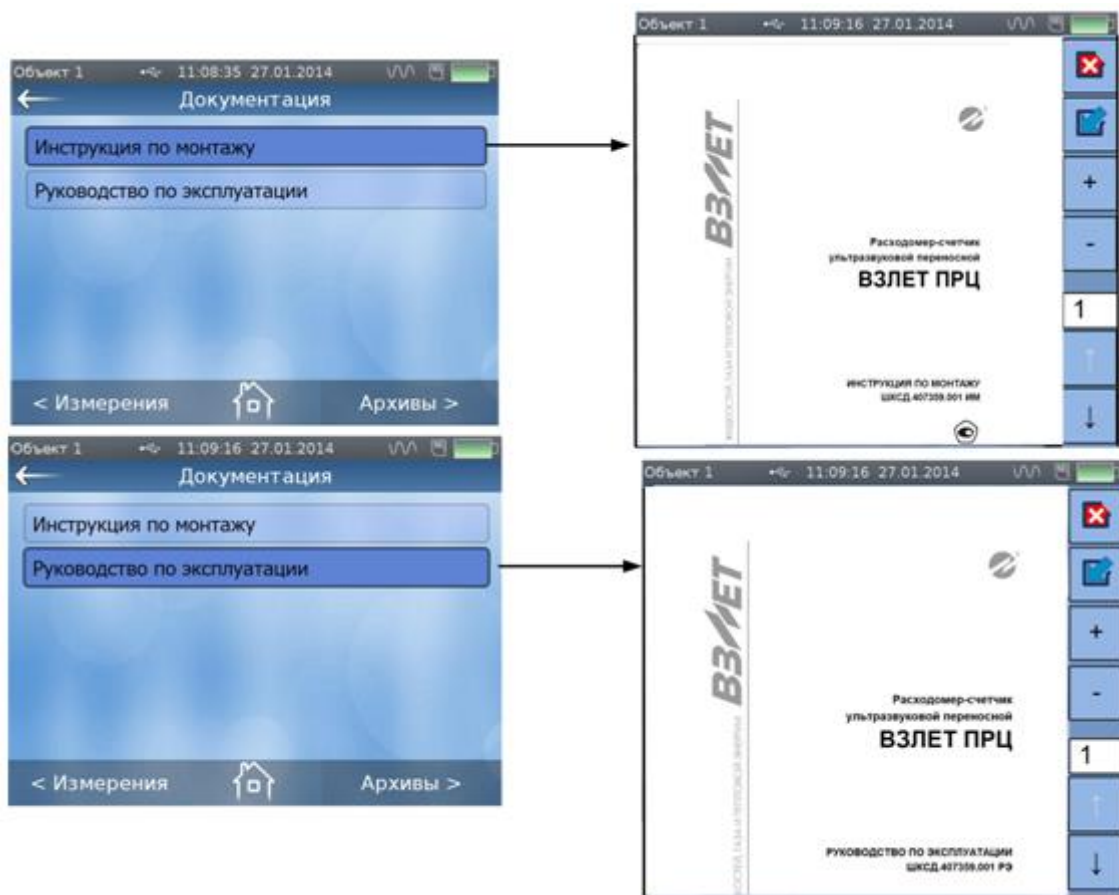
Рис.18. Окно «Документация».
