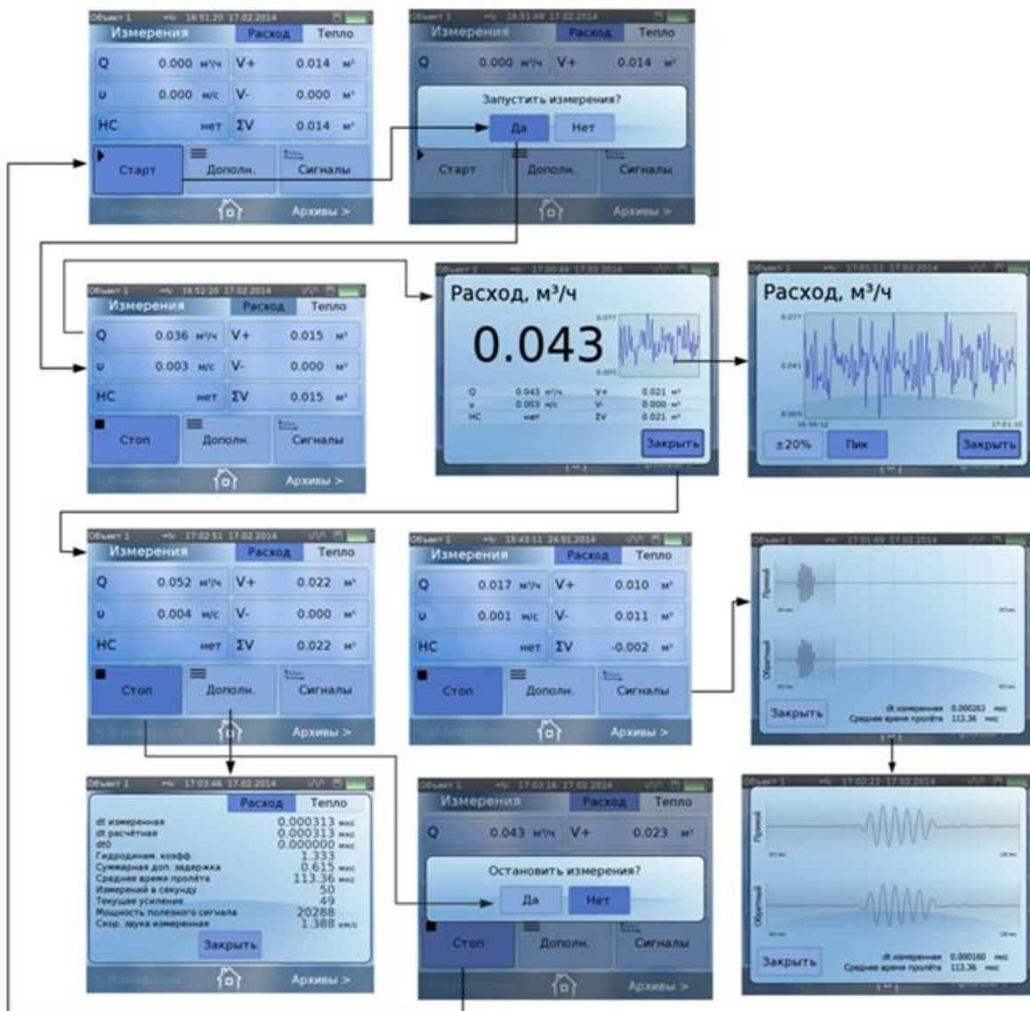
Рис.13. Окно «Измерения / Расход».
