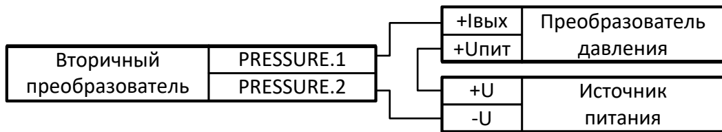
Возможная схема подключения датчика давления
