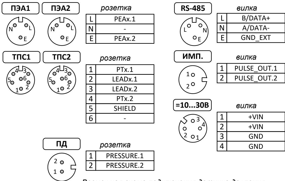
Возможная схема подключения датчика давления
