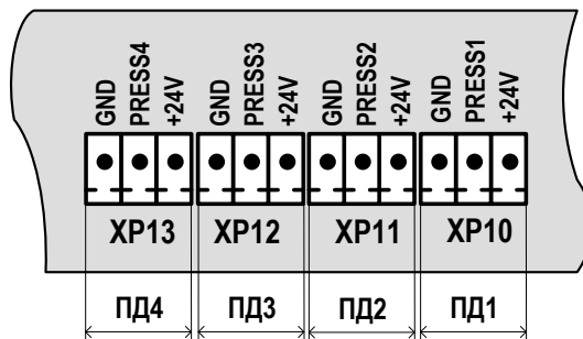
Рис.10. Обозначение коммутационных элементов подключения ПД.
