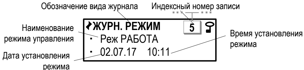
Рис.15. Вид окна индикации «Журнала режимов».
