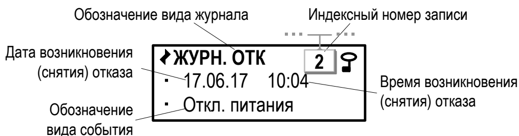
Рис.13. Вид окна индикации «Журнала отказов».
