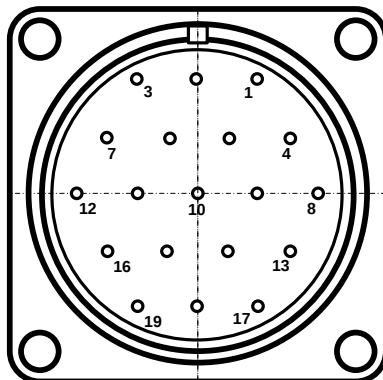
Рис.В.1. Разъем питания и связи
