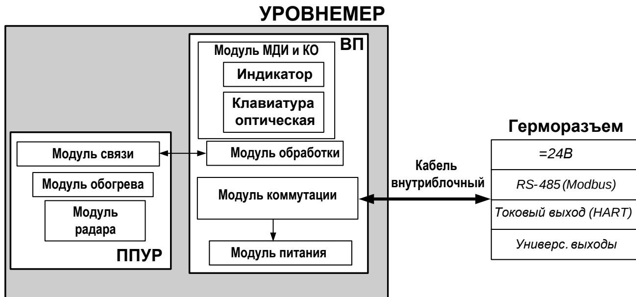
Рис.2. Структурная схема уровнемера.
